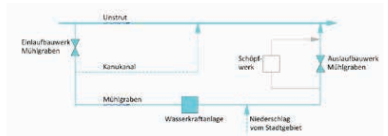
Funktionsprinzip der Wasserführung von Unstrut, Mühlgraben und Kanalkanal bei Normalwasserstand der Unstrut.
