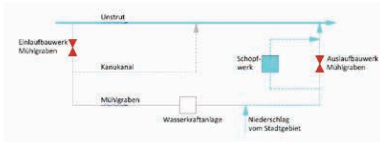
Funktionsprinzip der Wasserführung von Unstrut, Mühlgraben und Kanukanal bei Hochwasserstand der Unstrut. Quelle Grafiken: ICL Ingenieur Consult GmbH, Leipzig
